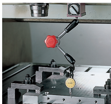
M/Cでの使用
