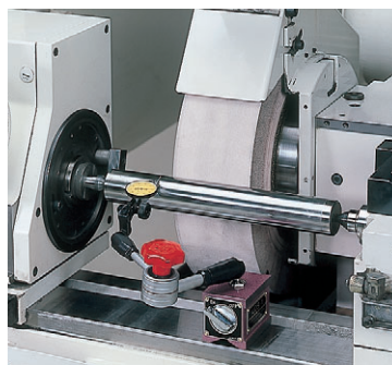
研磨機での使用
