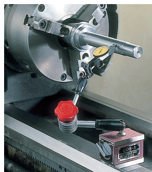
NC旋盤での使用
